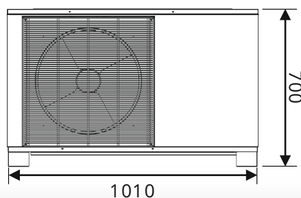
venkovní jednotka SPLITplus-6
